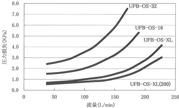
UFB-OS-シリーズ 圧力損失グラフ
