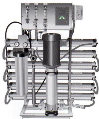
RO(逆浸透膜)装置 純水装置
